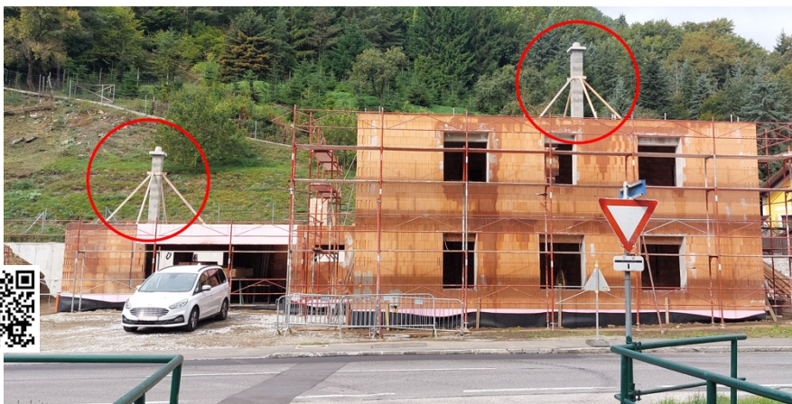
AHRENS Abgassysteme mit Abstützung bis zur Versetzung des Dachstuhles.
