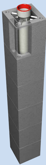
BÜ-Überdruckabgasleitung
