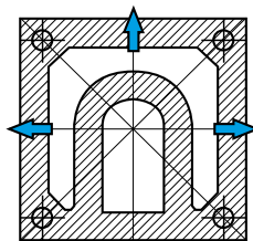
Unterer LIV-Sockelstein
